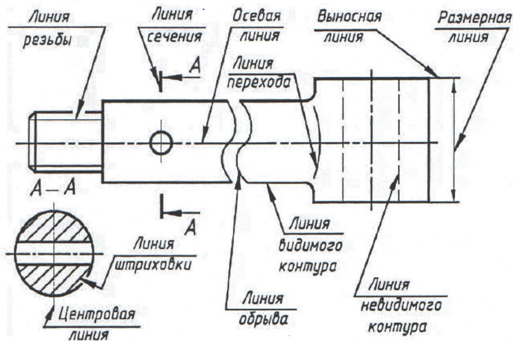
Рис. 4. Примеры выполнения линий чертежа
